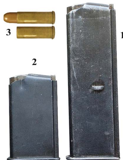
1. сменный коробчатый магазин на 20 патронов 7,63 мм; 2. сменный коробчатый магазин на 10 патронов 7,63 мм; 3. французский патрон и гильза 8х27 мм Mle.92
